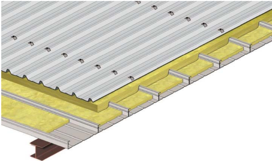
Figure 1 Couverture double peau à trame croisée sur plaque nervurée et plateau
