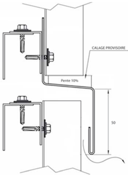
BAVETTE DE RACCORD INTERMÉDIAIRE ÉPAISSEUR = 1 mm R. INT = 3 mm
