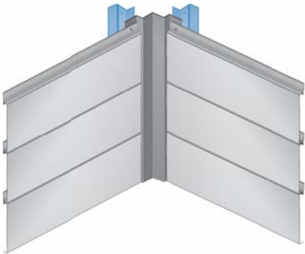
Détails d'angle
