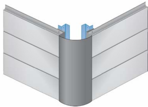
Détails d'angle
